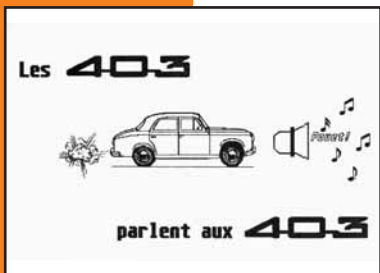
cpClu.1
