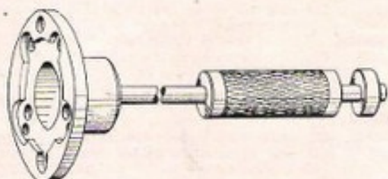
Extracteur de moyeu AV et d'arbre de roue AR Fenwick 8.0501
