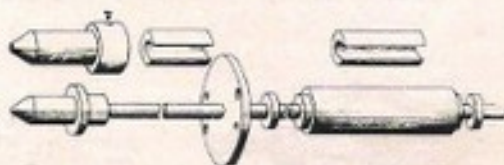
Appareil pour remontage du roulement milieu arbre transmission Fenwick 8.0403
