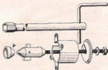
Extracteur de roulement d'arbre de transmission Fenwick 8.0402
