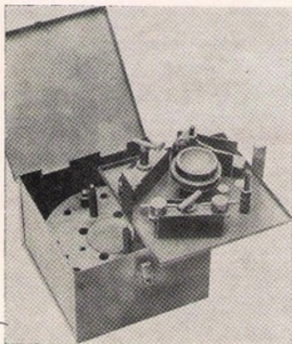
Coffret d'outillage pour pont AR Fenwick 8.0505
